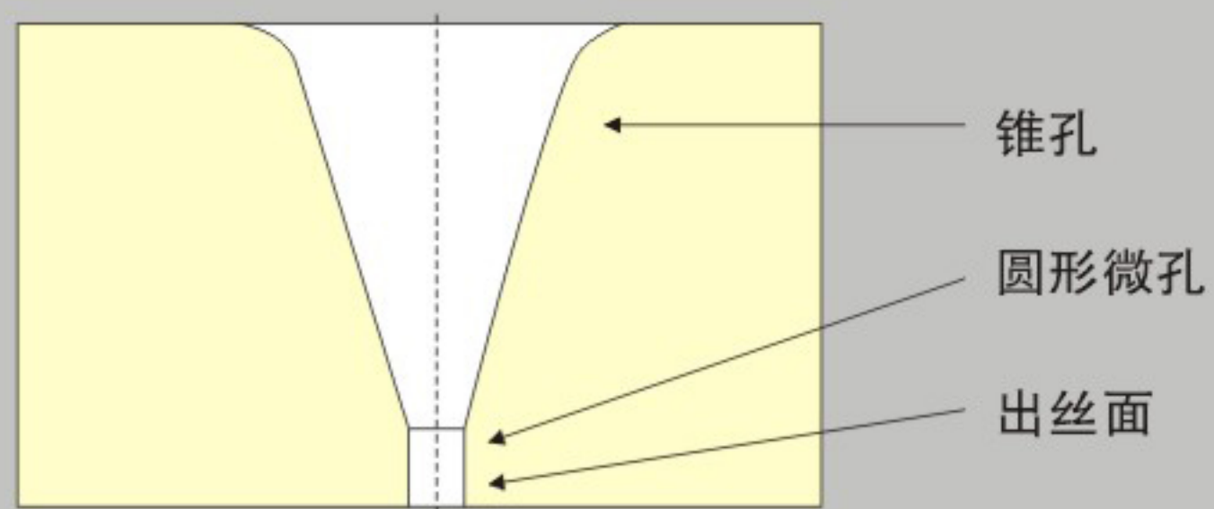
湿纺喷丝头孔形
