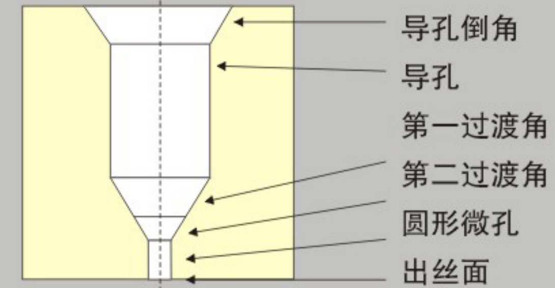
溶纺喷丝板孔形
