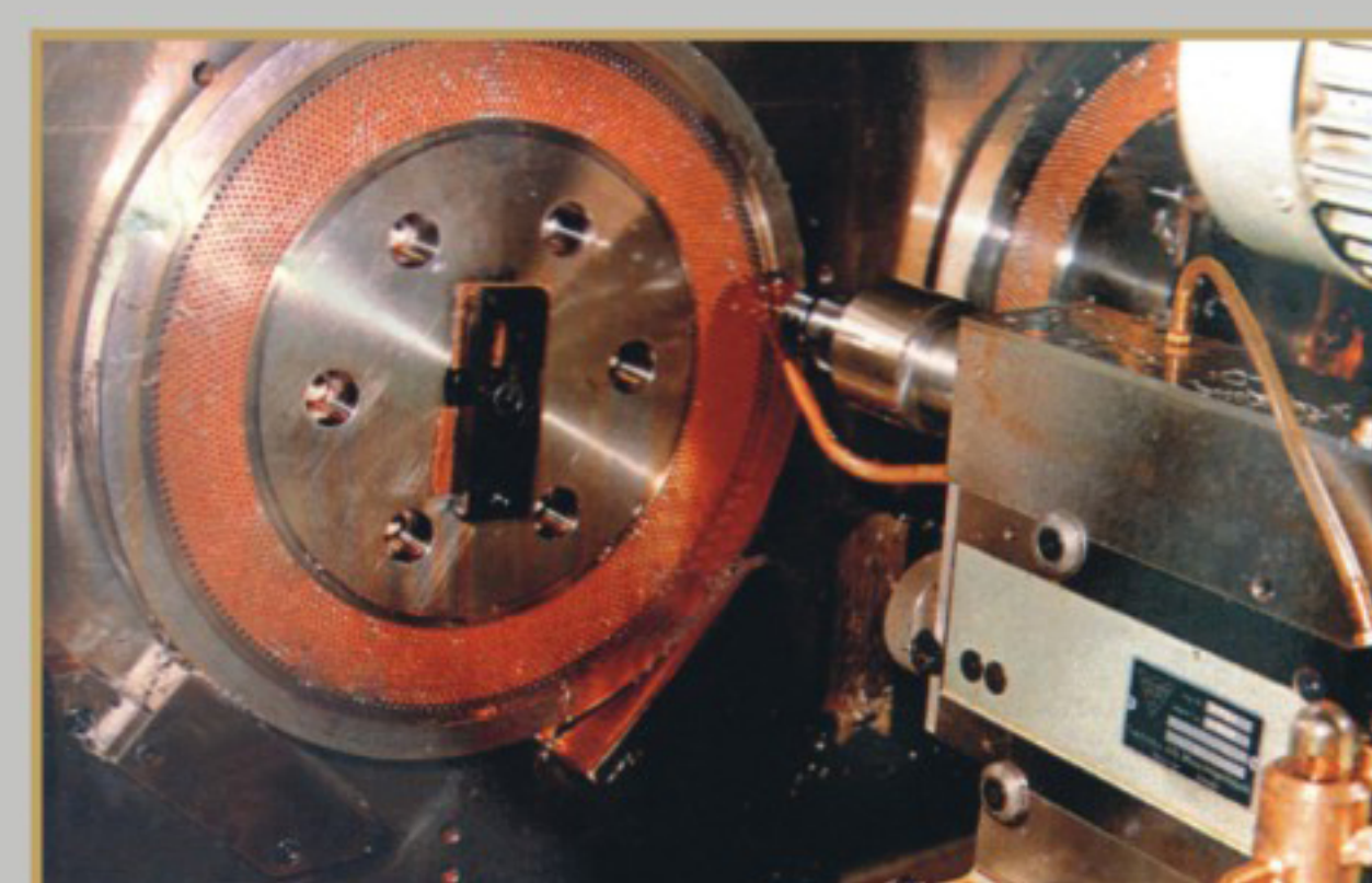
喷丝板加工 Spinneret machining
